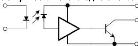
Электрическая схема одного канала
