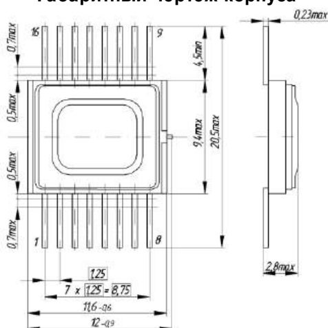
Габаритный чертеж корпуса
