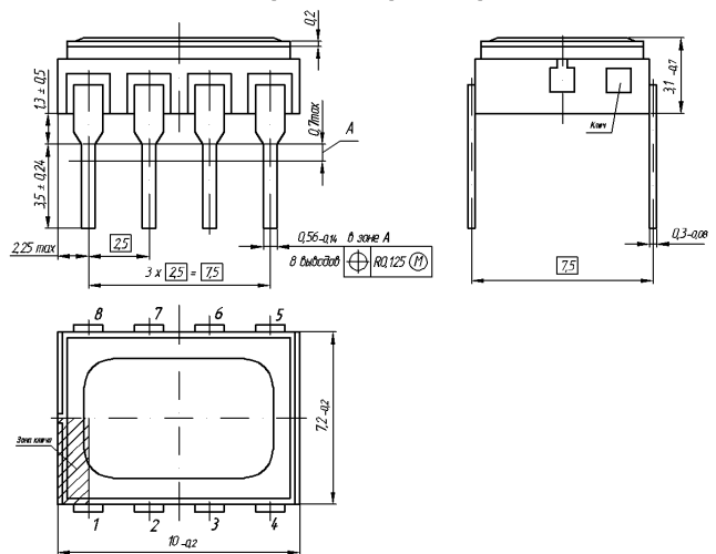
Габаритные размеры
