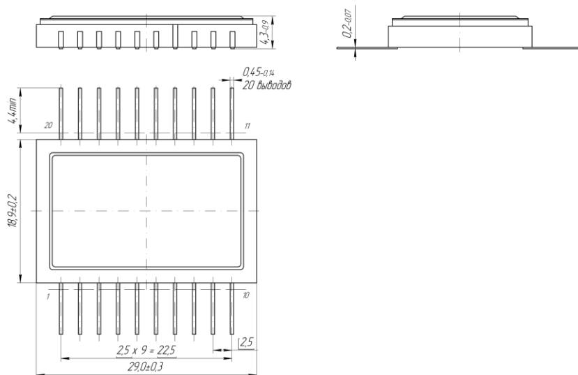
Рисунок 1 – Общий вид и расположение выводов микросборок
