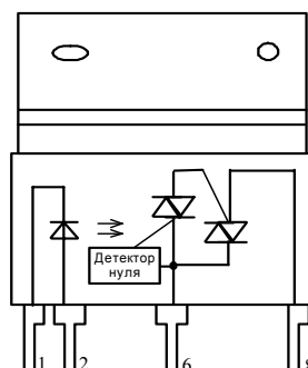
К450КП1
