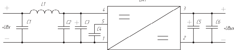
Схема применения
