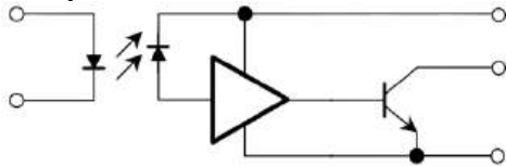
Электрическая схема одного канала
