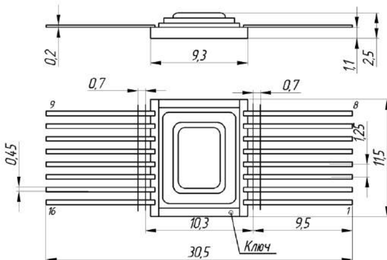
Габаритные размеры
