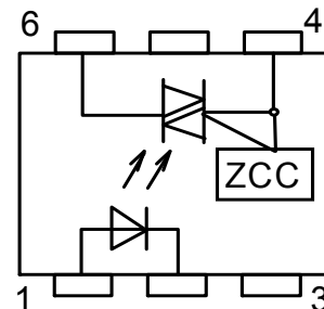
Электрическая схема
