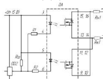
Схема В:
