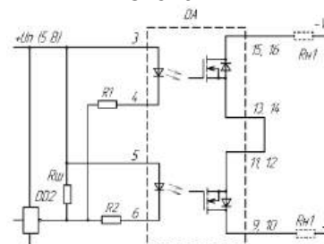
Схема В:
