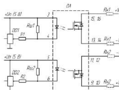
Схема Б:
