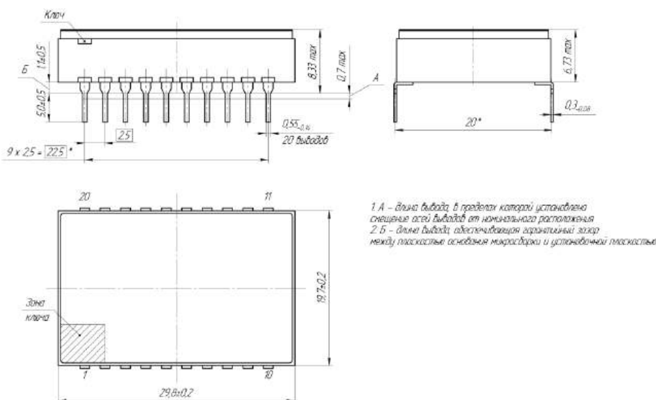
Габаритный чертёж корпуса
